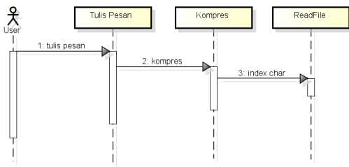
Gambar 16 Sequence Diagram Kompresi Pesan
