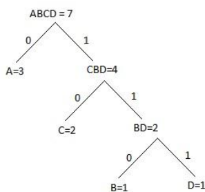
Gambar 1 Pohon Huffman Untuk Pesan ABACCDA
